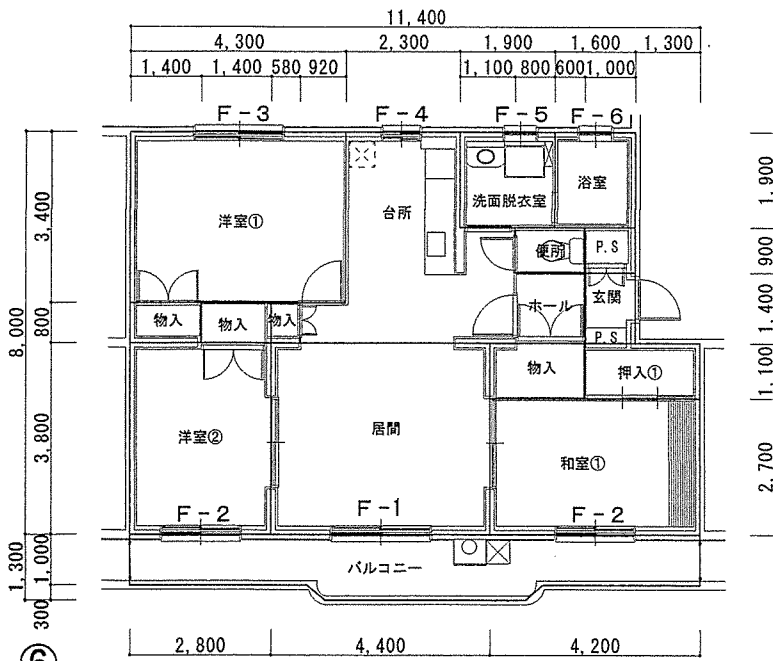
⑥ 第4宿舎203号棟(タイプd)標準平面図
