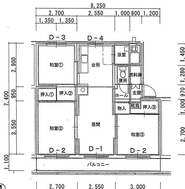
第4宿舎201号棟標準平面図
