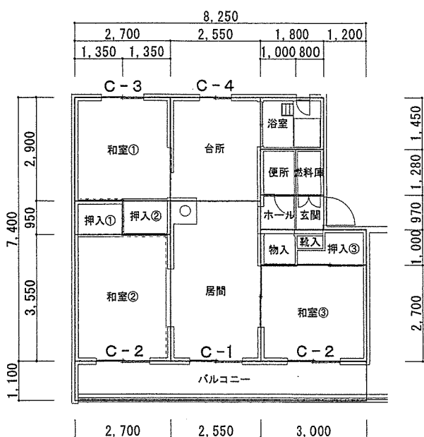
第4宿舎200号棟標準平面図
