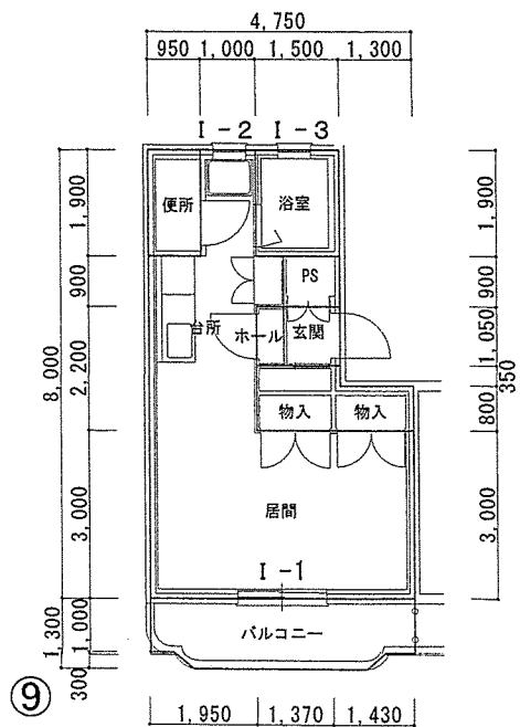
⑨ 第4宿舎204号棟(タイプa)標準平面図
