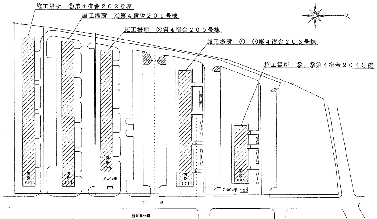
第4 宿舍建物配置図 S=1 : X
