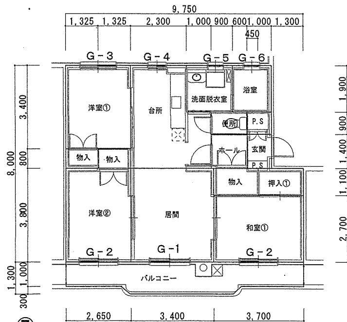
⑦ 第4宿舎203号棟(タイプc)標準平面図
