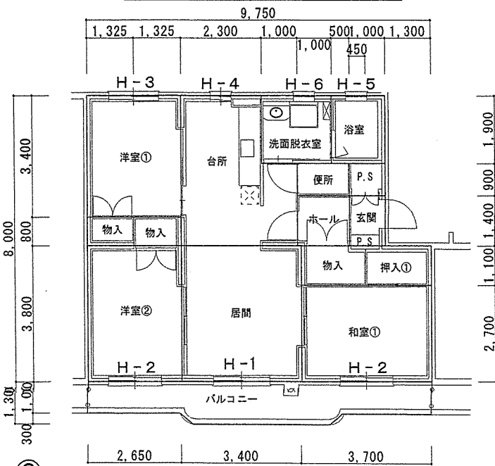
⑧ 第4宿舎204号棟(タイプc)標準平面図
