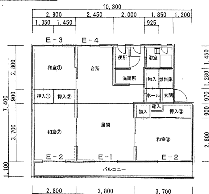
第4宿舎202号棟標準平面図
