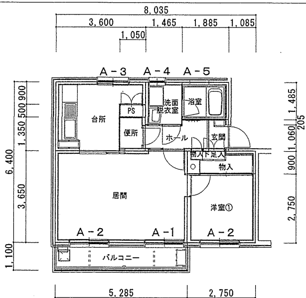
第1宿舎5号棟標準平面図
