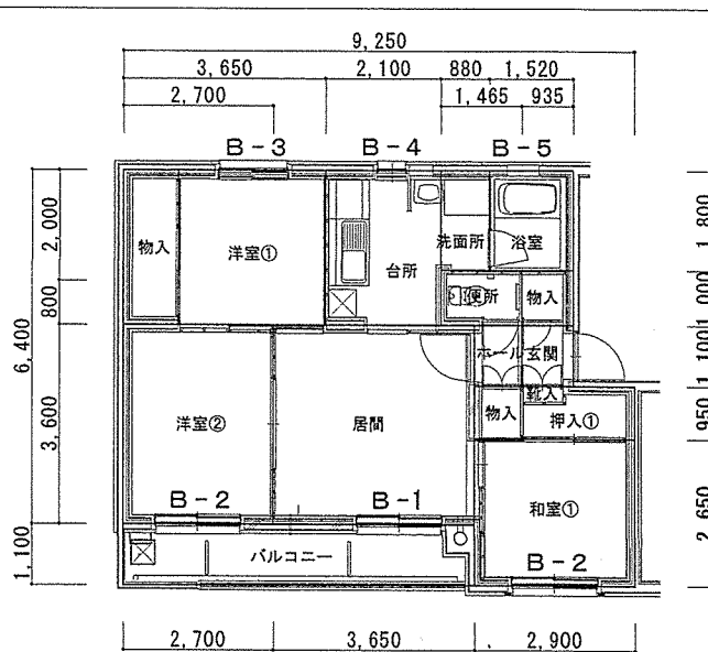
第1宿舎6号棟標準平面図
